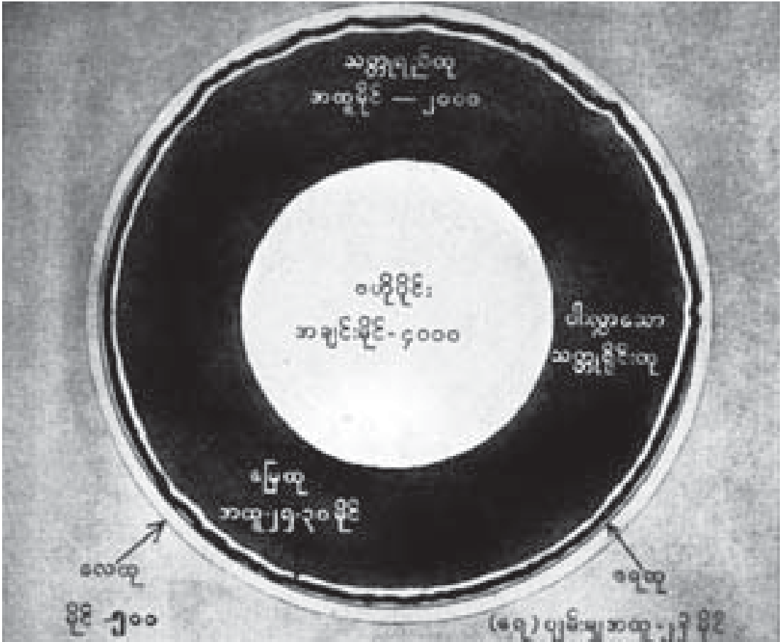
သိပ္ပံပညာအလိုအရ ကမ္ဘာတွင်အထပ်ကြီး ၆ ထပ်ပါဝင်သည်။ အတွင်းကျဆုံးဗဟိုဝိုင်းကို သံနှင့် နစ်ကယ်သတ္တုရည်ထူက ဝန်းရံထားသည်။ အပေါ်ဆုံးအထပ်မှားမူ မြေထုပင်ဖြစ်သည်။
