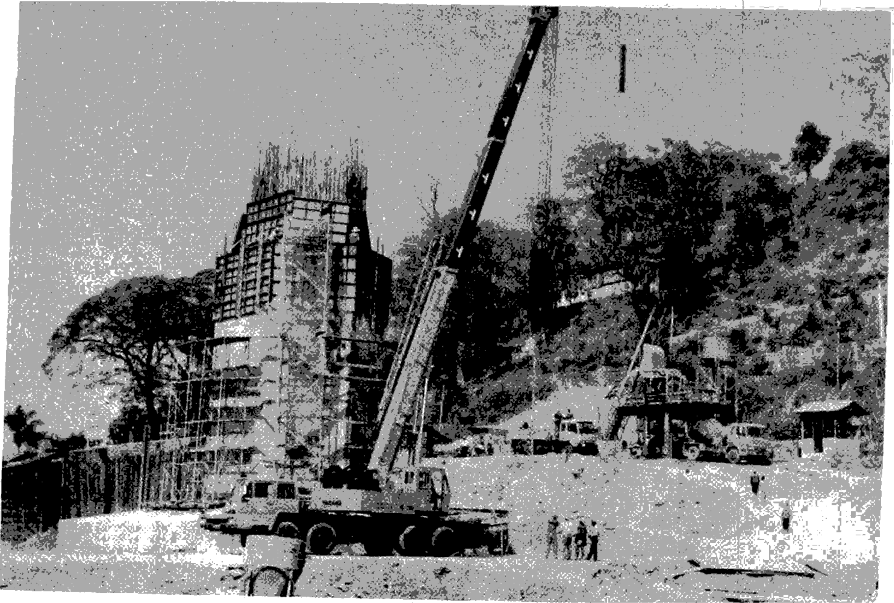
ဧရာဝတီတံတား (ပြည်) ရေလည်တိုင် အမှတ်(၁) ကွန်ကရစ်လောင်းရန်ပြင်ဆင်ခဲ့စဉ်က
