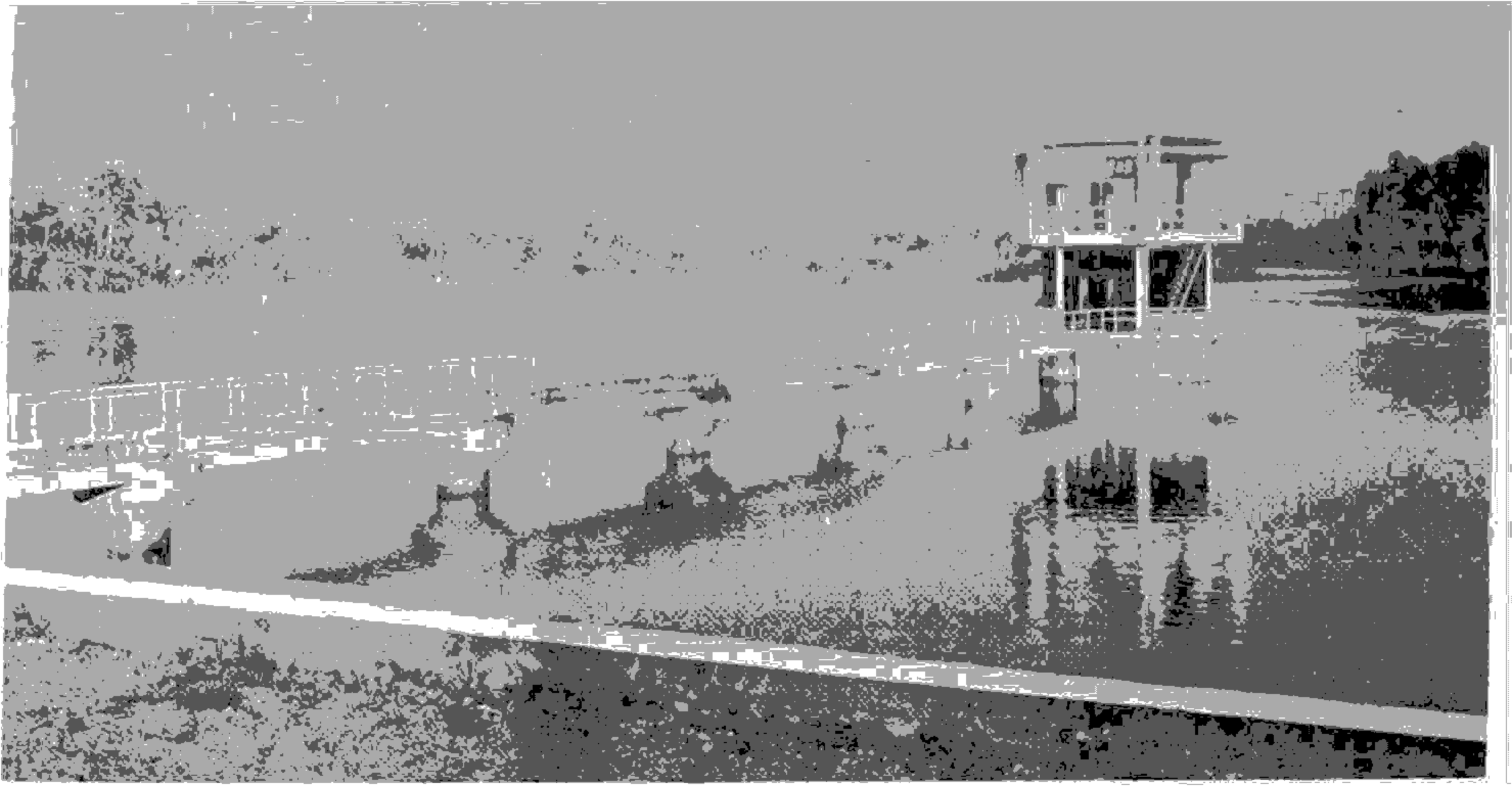
တိုက်ကြီးမြို့နယ် ဥက္ကံချောင်းပေါ်တွင် တည်ဆောက်ခဲ့သော တဘူးလှ (ဥက္ကံ) ရေလှောင်ကန်၊ ရေထိန်းမျှော်စင်နှင့် တံတား
