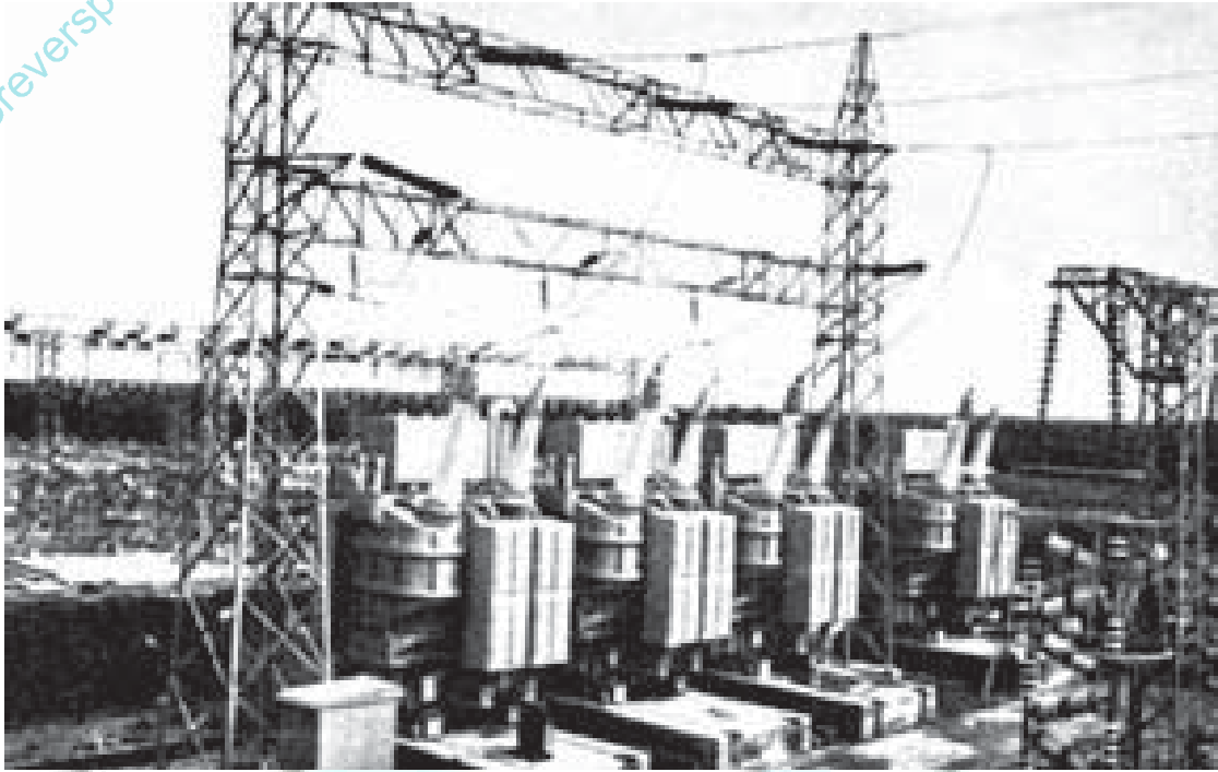
လောပီတမုရရှိသော လျှပ်စစ်ဓာတ်များကို တဆင့်ပို့ပေးရသော ကေမီ၊ အေ ၆၀,၀၀၀ အားရှိသည့် ဓာတ်အားဖြန့်စက်ကြီး
