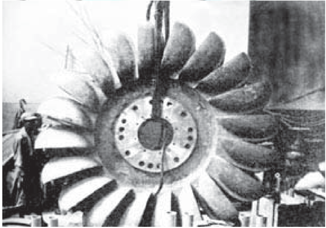
ရေအားမှ လျှပ်စစ်ဓာတ်အားအဖြစ်သို့ ပြောင်းလဲပေးမည့် ရေဟုတ်ကြီးတင် ခွက်ကြီးများ ပါရှိသည်။ ပန်းထွက်လာသော ရေအဟုန်သည် ထိုခွက်ကြီးများကို အရှိန်ပြင်းစွာ တန်းသဖြင့် ရဟုတ်ကြီး လည်ရခြင်းဖြစ်သည်။
