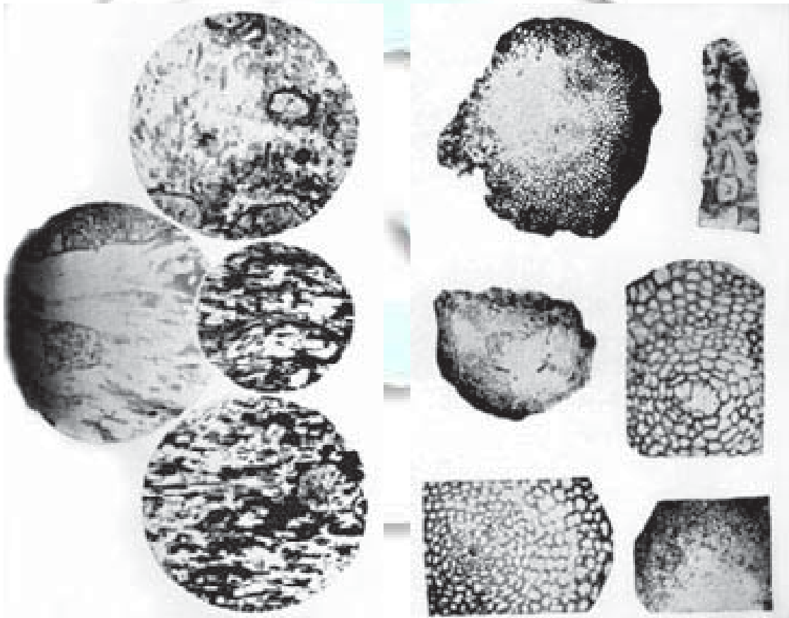
လွန်ခဲ့သောနှစ်သန်းပေါင်း ၅၀ခန့်က ဖြစ်ပေါ်ခဲ့သော ထုံးကျောက်လွှာများအတွင်းရှိအဏုရုပ်ကြွင်းကျောက်များ၏ဖြတ်ပိုင်းပုံ။အဏုရုပ်ကြွင်းကျောက်များကို လေ့လာသော ပညာမှာ အဏုနိခါတကဗေဒ ဖြစ်၍၊ ရေနံမြေဒေသရှိ ကျောက်လွှာများ ပြန်လှန်ဆက်စပ်ရေးတွင် အထူး အသုံးဝင်သည်။
