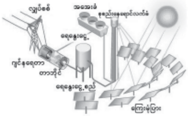
စုစည်းနေရောင်အပူနည်းပညာ
